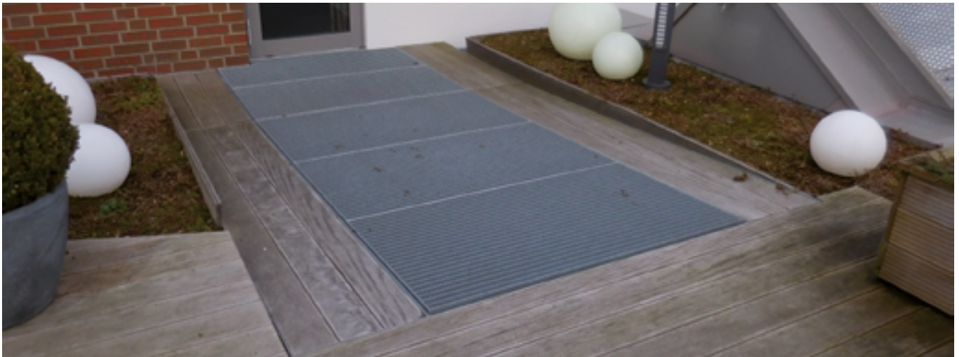
Bei Hoteleingängen sollten eingearbeitete Gitterroste statt Rasenteppiche oder Fußmatten verwendet werden.
