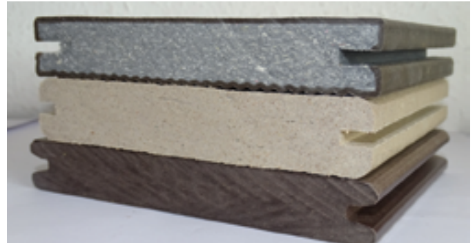
Vollprofile sind vorwiegend komplett durchgefärbt, bei co-extrudierten Profilen kann der Kern farblich unterschiedlich sein.
