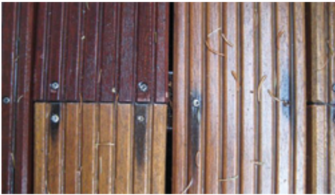
Gerbsäure von Bangkirai hat mit den Schrauben reagiert. Die Verfärbung ist kaum noch zu beseitigen.
