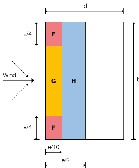
Einteilung der Flächen ( e = b oder 2h )
