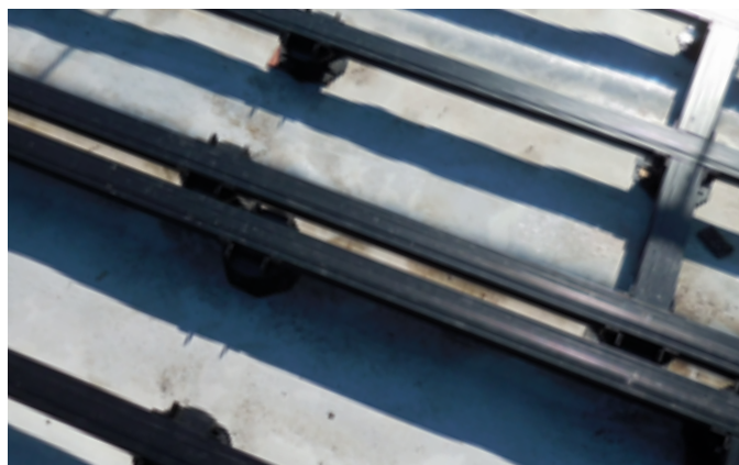
Aluminiumunterkonstruktion werden oftmals mit Verstellfüßen als System angeboten und müssen nur eingeklickt werden.
