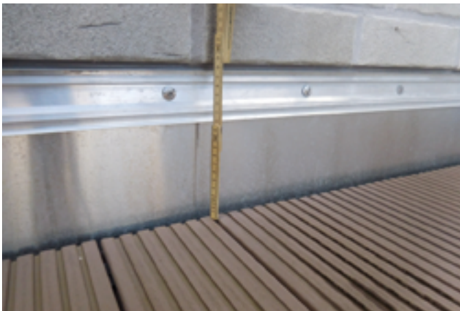
Die Abdichtung sollte am Gebäude min. 150 mm über die Oberfläche der Terrasse geführt werden und ist z. B. mit Verbundblechen oder Klemmprofilen zu sichern.
