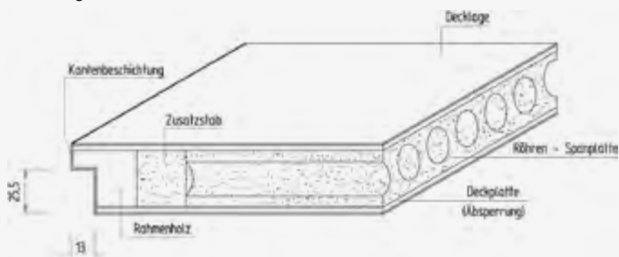
Innenleben einer Röhrenspanptür
