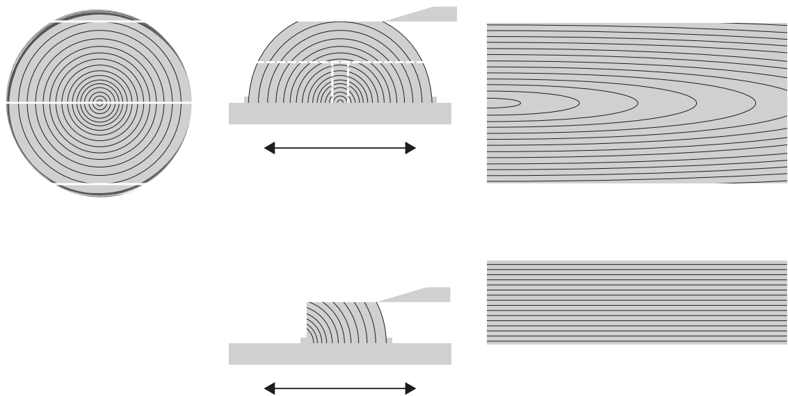
Herstellung und Furnierbild Schäl furnier
