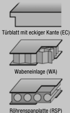
Röhrenspanplatte (RSP)
