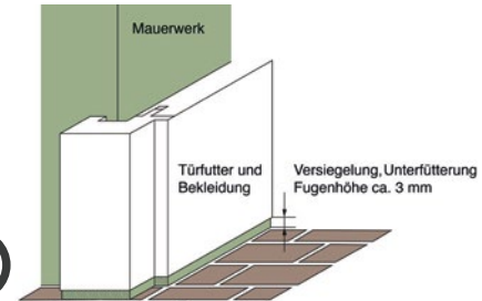
Unterer Anschluss bei nicht saugfähigen Untergründen
