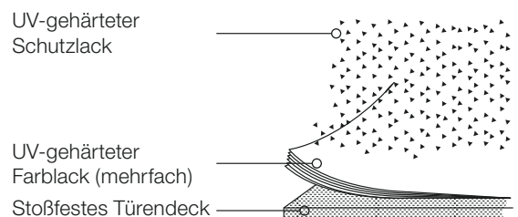
Beschichtung mit Lacksystemen
