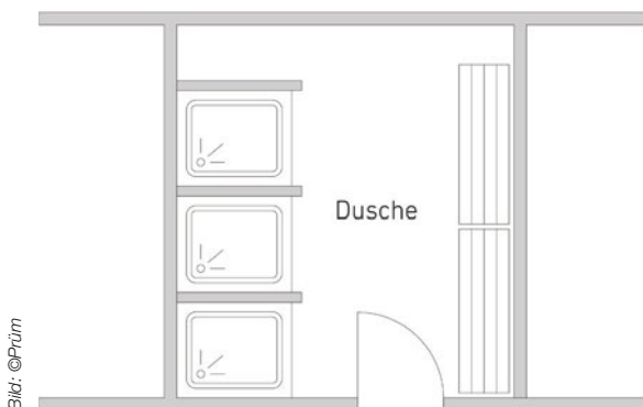
Beispiel für den Einbau einer Nassraumtür. Die Tür führt in einen Raum, in dem mit hoher Luftfeuchtigkeit und ständigem Spritzwasser zu rechnen ist.
