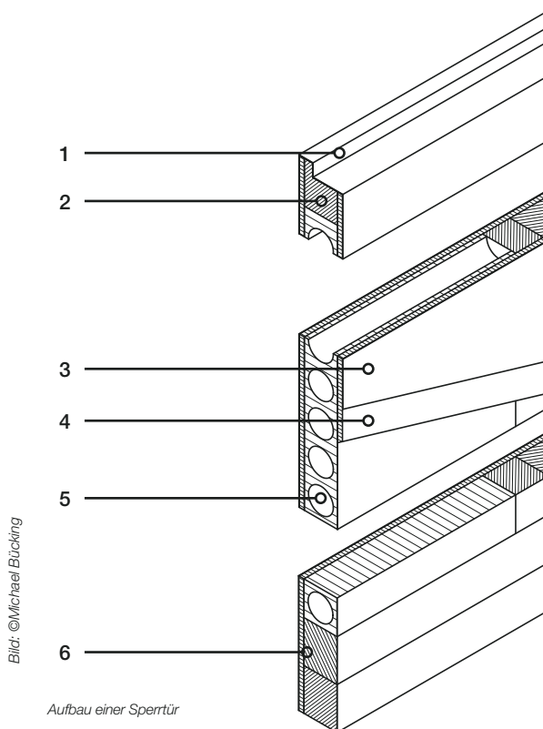
Innenleben einer Röhrenspanstreiftür
