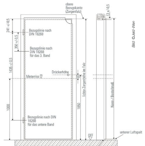
Positionierung der Drücker und Bänder
