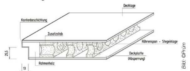
Innenleben einer Röhrenspanstreiftür
