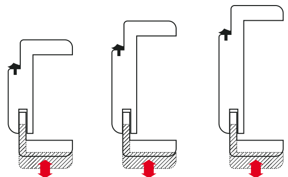
Verstellbereich Umfassungszarge
