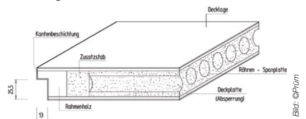
Innenleben einer Röhrenspantür
