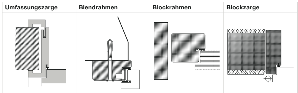
Konstruktionsarten Türrahmen und Türzargen
