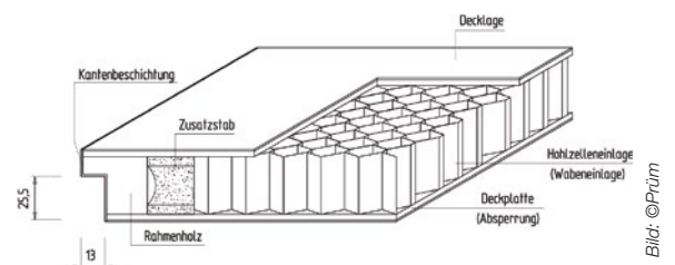
Innenleben einer Wabentür
