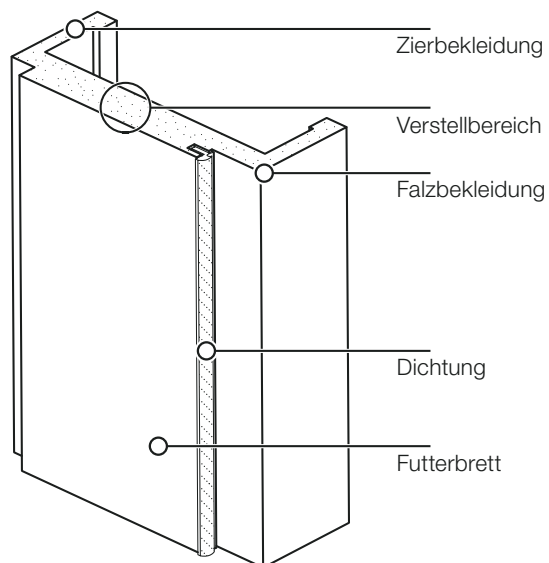
Konstruktionsdetails Umfassungszarge
