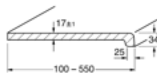
Profil Exclusiv
