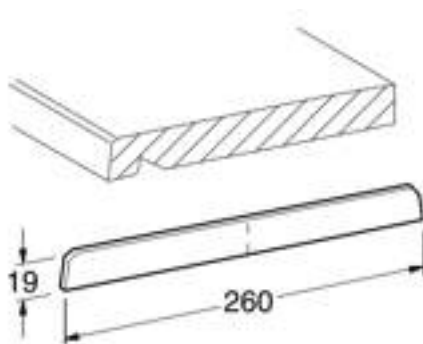
Seitenabschlusskappe 19/260 mm
