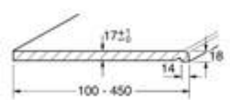
Profil Compact
